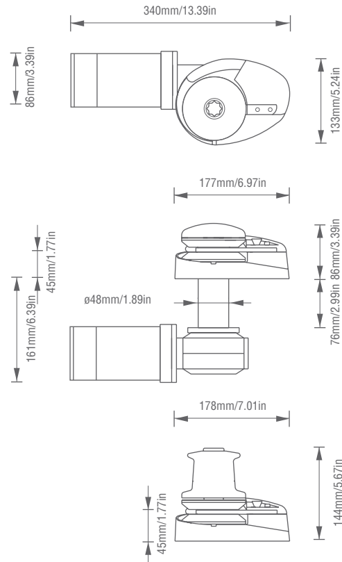
VRC 600
