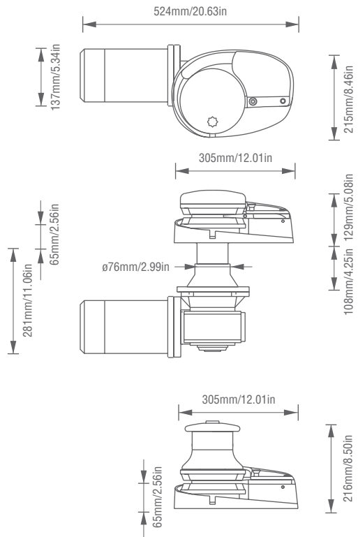
VR 2500/3500
