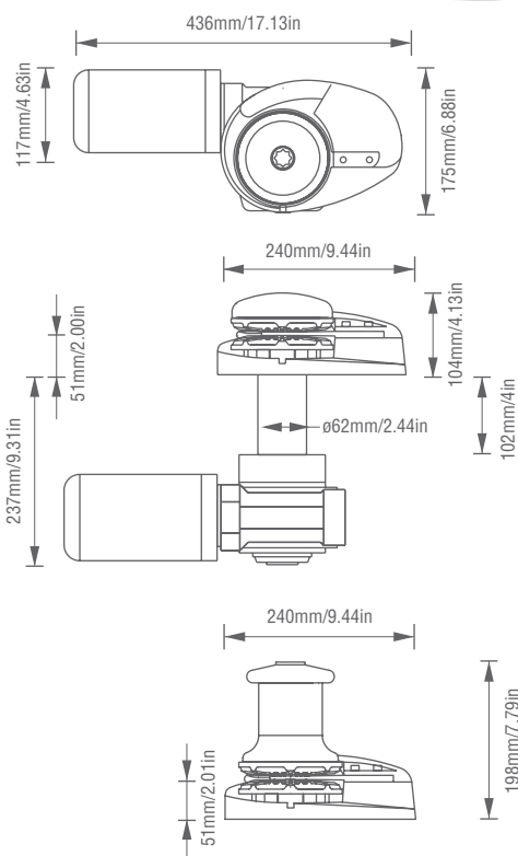
VR 1200
