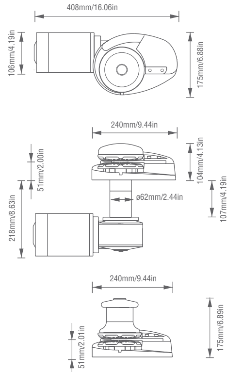
VRC 1000
